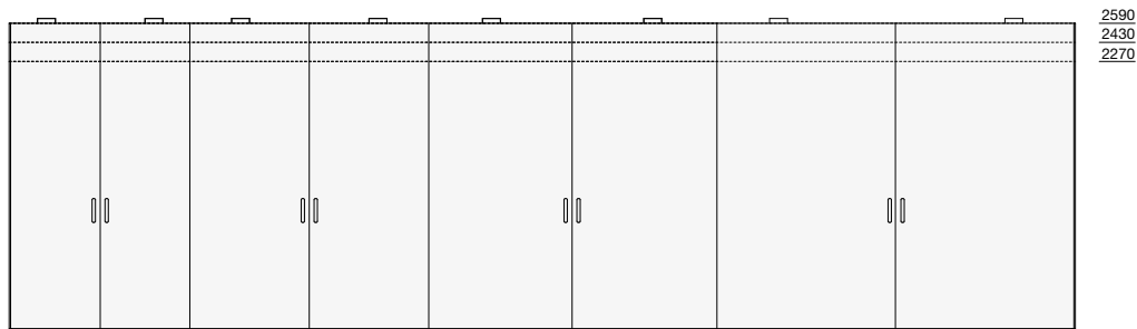
Altezze e prospetti moduli con ante Modules with doors - height and front view
