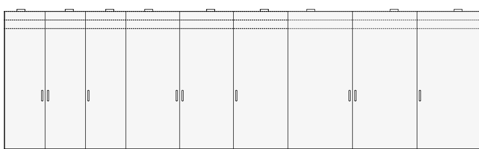
Altezze e prospetti moduli con ante Modules with doors - height and front view
